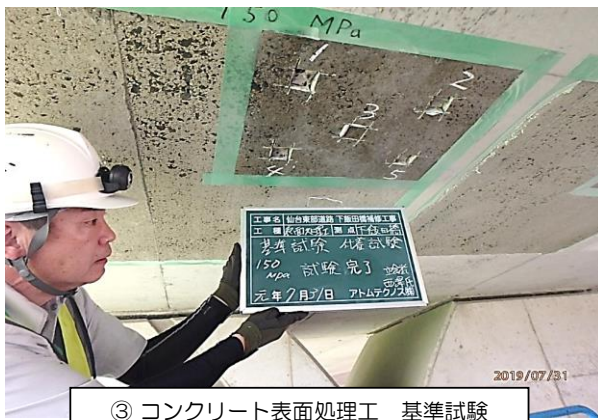
③ コンクリート表面処理工 基準試験
